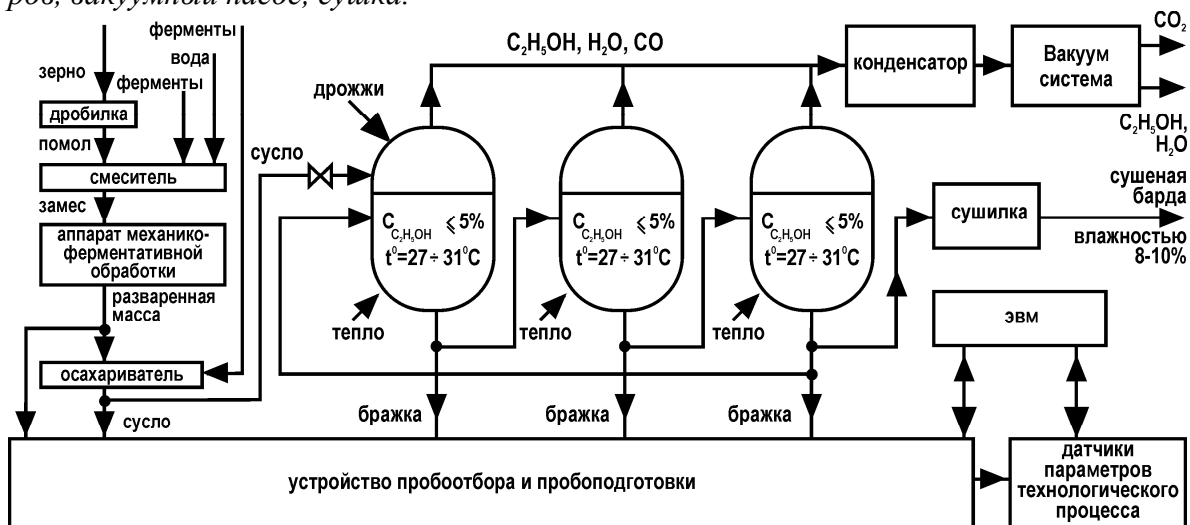
Рис. 1 Функциональная схема установки для комплексной переработки зерна на спирт и кормопродукты
